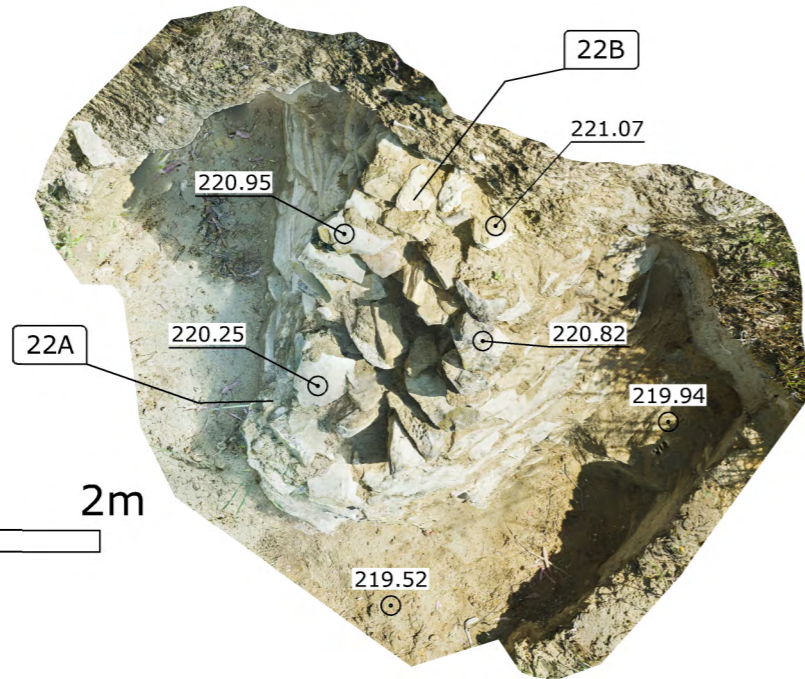
Muro bajo ladera. Planta
